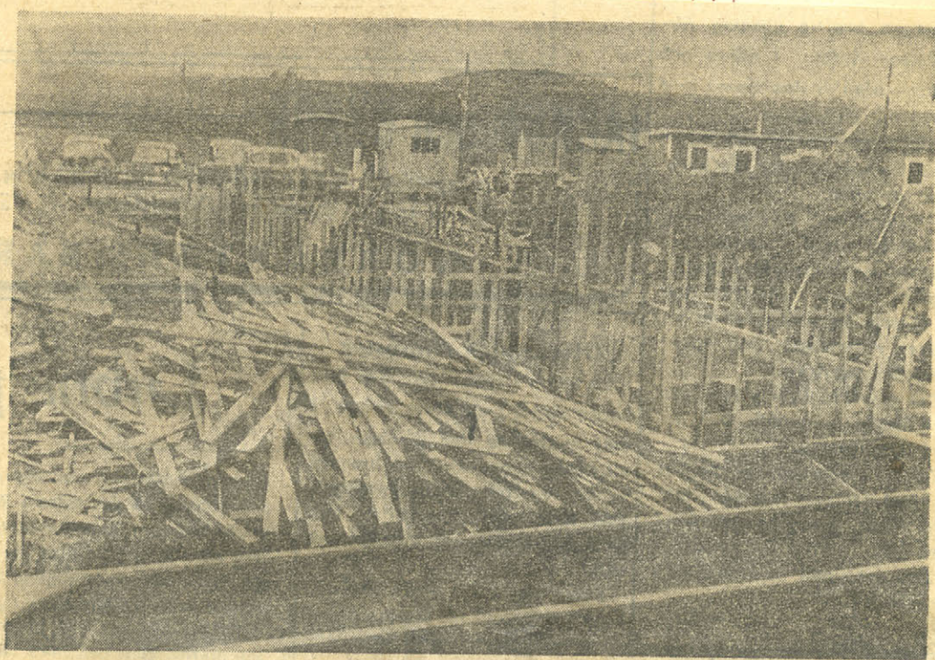
Här ses förluftnings- och sedimenteringsbassängen under uppförande
