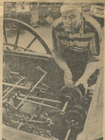
Växelhjulen är fyndigt konstruerade, säger hr Almkvist. Backväxeln är betydligt mer lågväxlad än de två framåtgående växlar. Låter man så ångmaskinen köra baklänges, kan man utnyttja denna "krypväxel" för framåtdrift.
