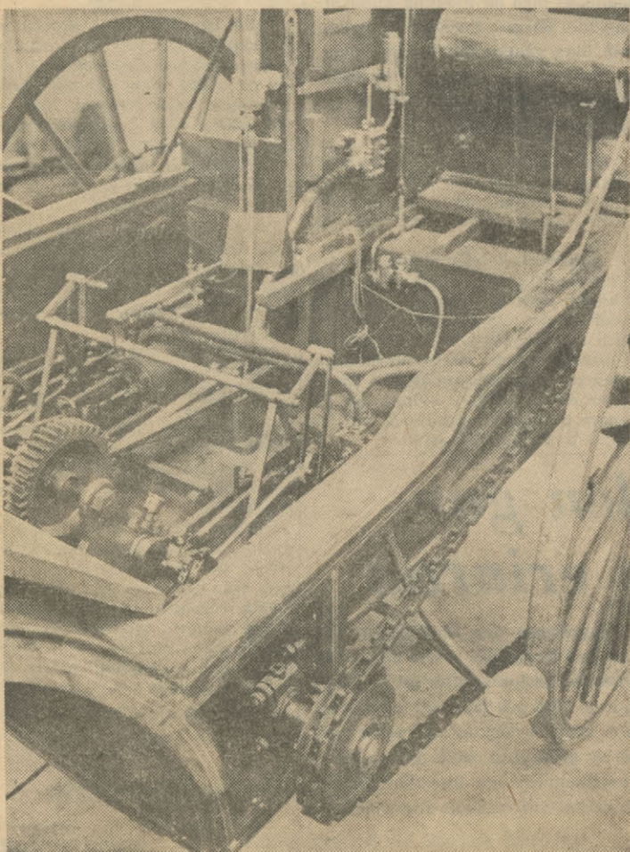
Nästan ett underverk av teknik. På vagnen finns det frikoppling, tre växlar, varvräknare, back, enhjulsdrift om så önskas och nästan ljudlös gång.
