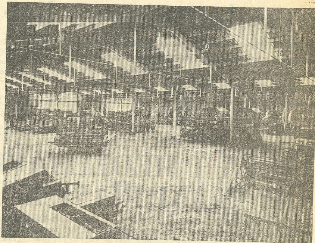
Maskinlagret omfattar 5.000 kvm och har fri takhöjd även för de största maskiner.
