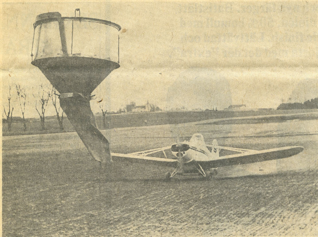
I förgrunden behållaren med gödning som tappas i en behållare i flygplanskroppen
