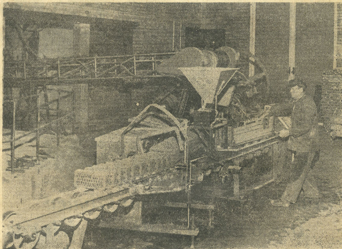
Maskin för helautomatisk tegeltillverkning.
