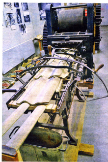
En av de maskiner från bruket som pressade takpannor. Med en speciell frångtagargaffel plockades pannorna från pressen.
