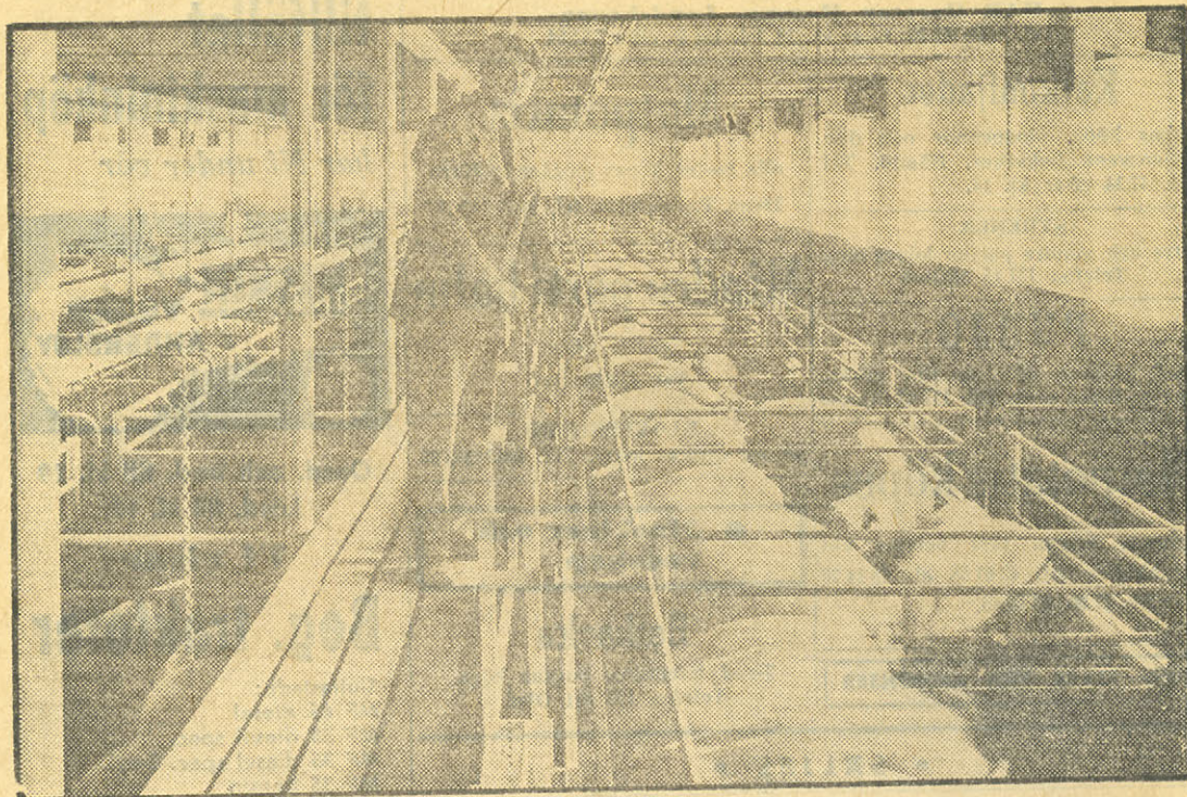
Förvaltare Stig Andersson prövar utfodringsanordningen i det högmekaniserade svinstallet.
