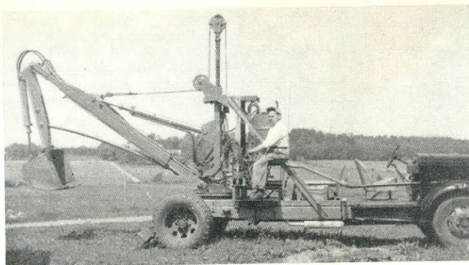
Den hemtillverkade svenska grävmaskinen på lastbilschassi.
