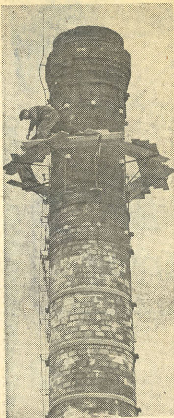
Erik Nilsson med hemort i Markaryd har bjudet skurupsborna på underhållning då han arbetar med tegelbrukets 40-meter höga skorsten som han gått över, med att laga i fogarna och sett över förbanden samt rivit ned fem meter av toppen då man nu håller på med att lägga in sugfläkt i skorstenen vilket gör att man kunnat kapa toppen.
