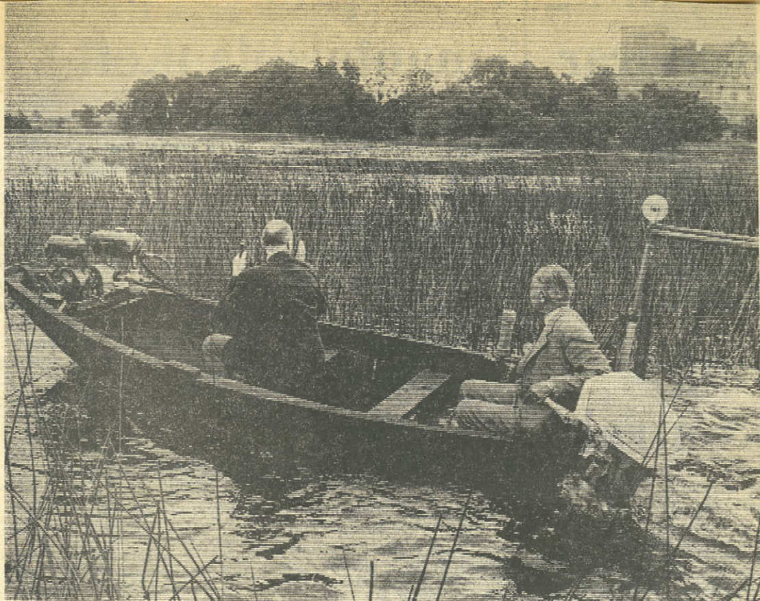
Hushållningssällskapets maskinkonsulent Sigfrid Andersson på ett av de rensningsaggregat som demonstrerades vid Svaneholmssjön. Vid rodet major C. T. Akrell, Smedstorp
