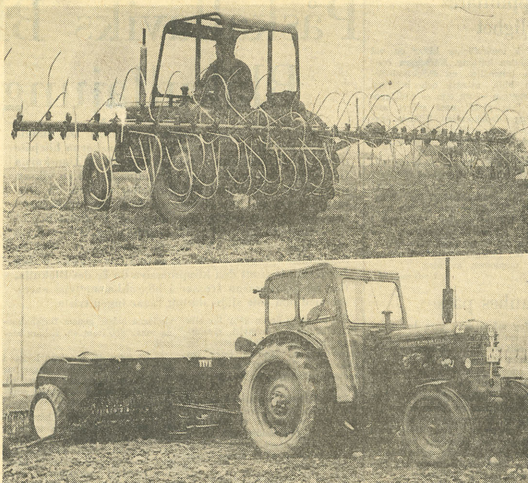
Överst Tives rullhöluckrare, en genialisk konstruktion utan mekanik, och därunder konstgödselspridaren SVC monterad framför sålådan på en såmaskin Tive H 5
