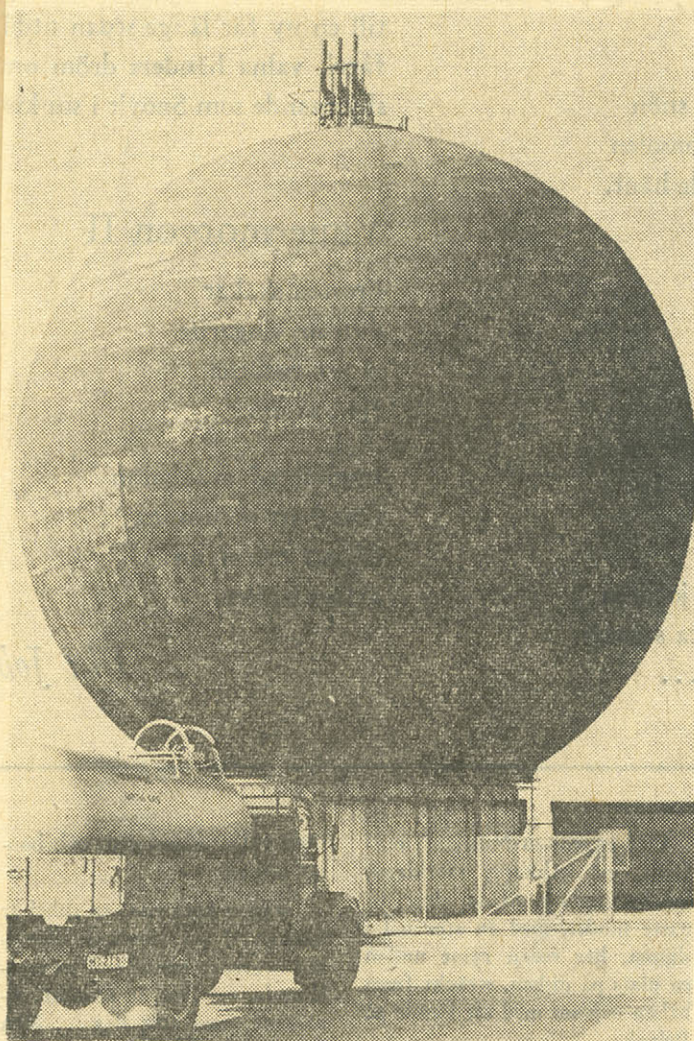
Med sin diameter på 22 meter och sin rymd av 3 000 ton är ammoniakkulan i Ystad ett originellt landmärke. Den skall så småningom målas i ljus färg.
