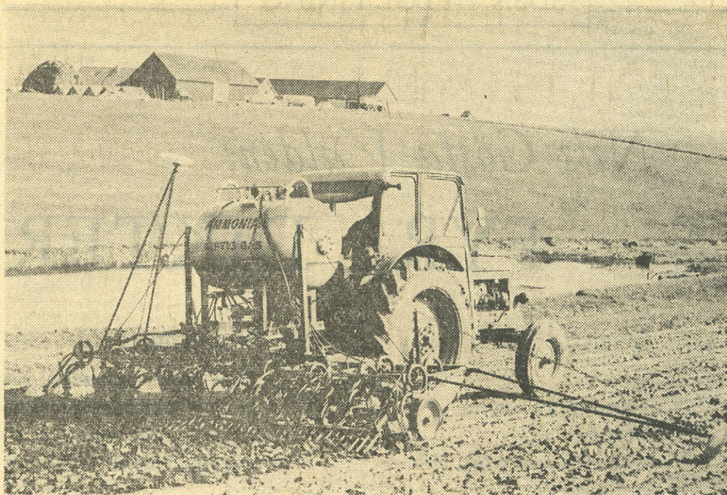
Marsk Stigs danska nedmyllningsaggregat i arbete på Sven Mårtenssons gård i Ullerup
