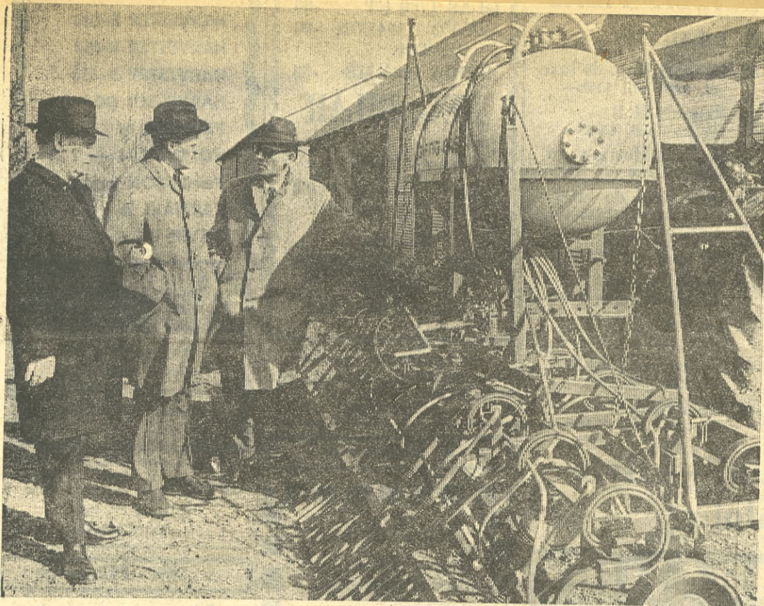
Nedmyllaren för ammoniak studeras här av riksdagsman Erik Grebäck och agronom Håkan Aldén, båda från Norsk Hydros svenska avdelning, samt ing. Jörgen A. Mortensen från Danmark. Maskinen är av dansk konstruktion och heter Marsk Stig.
