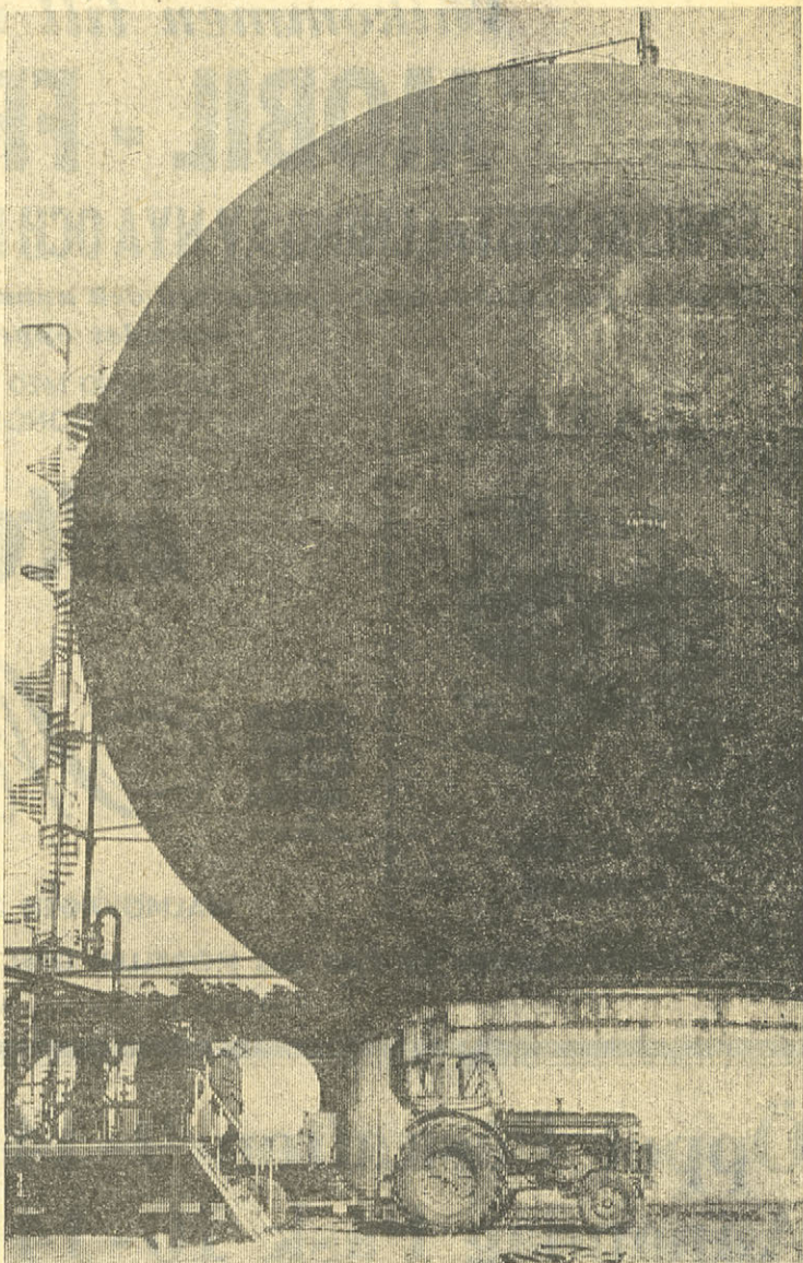
"Kulan" i Ystad rymmer 3.000 ton ammoniak. En transporttank från Jordberga gård fylls med 4 ton ammoniak på ca 10 minuter.
