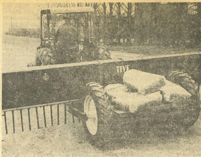
Konstgödselspridaren SVC monterad på en bärvagn, som kan ta 12 säckar. Obs! Gummirören slutar så nära marken, att vinden inte kan störa spridningen
