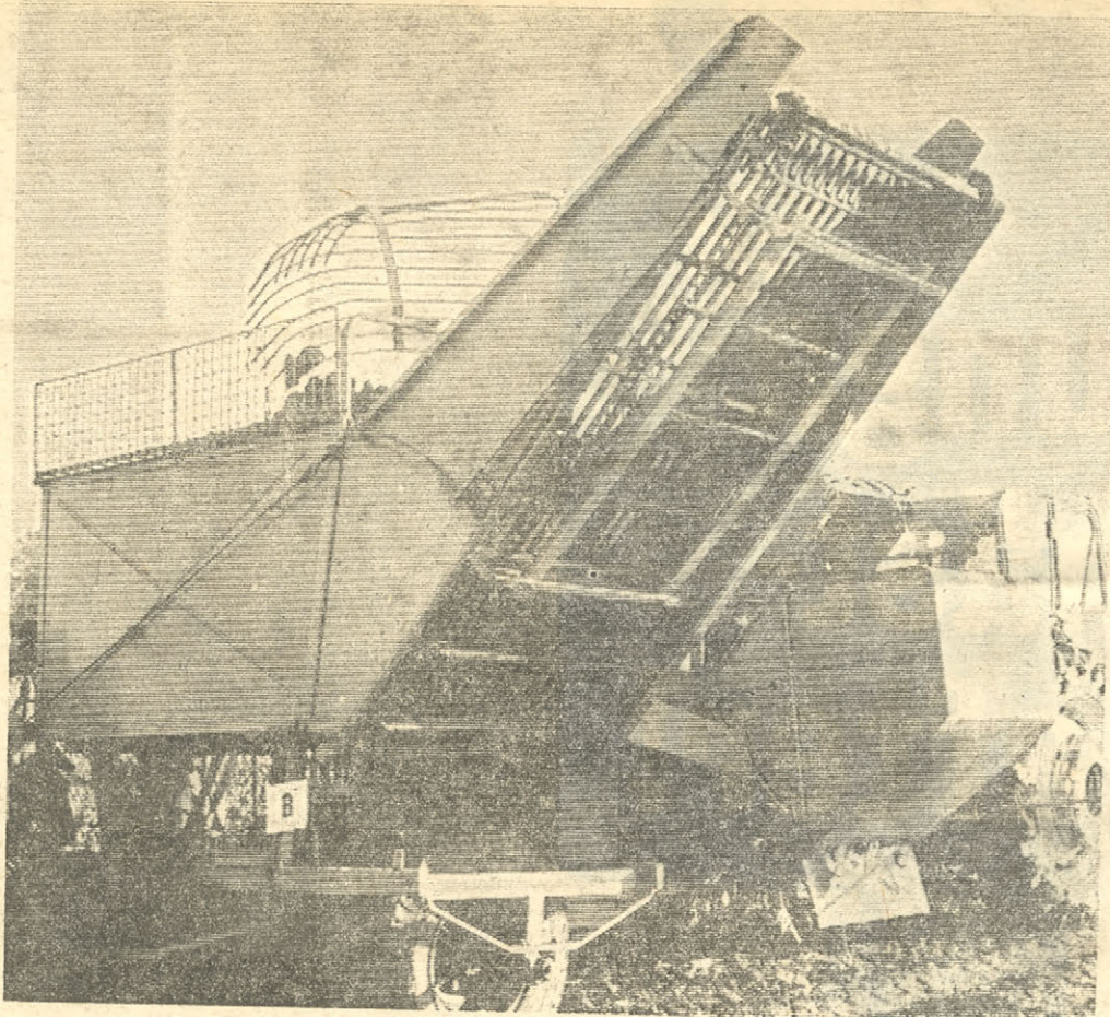
En av de danska maskinerna var Rational E-1A, en enradig helautomatisk betskördemaskin.
