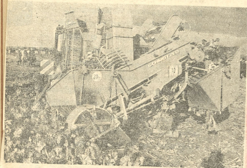
Tysktillverkade Schmotzer BK 2 var en enradig bogserad kraftuttagsdriven maskin, som tilldrog sig intresse.
