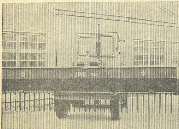
Tive SVCV spridare med radmyllningsaggregat.
